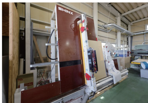
パネルソーHP-3シナックス3000A
